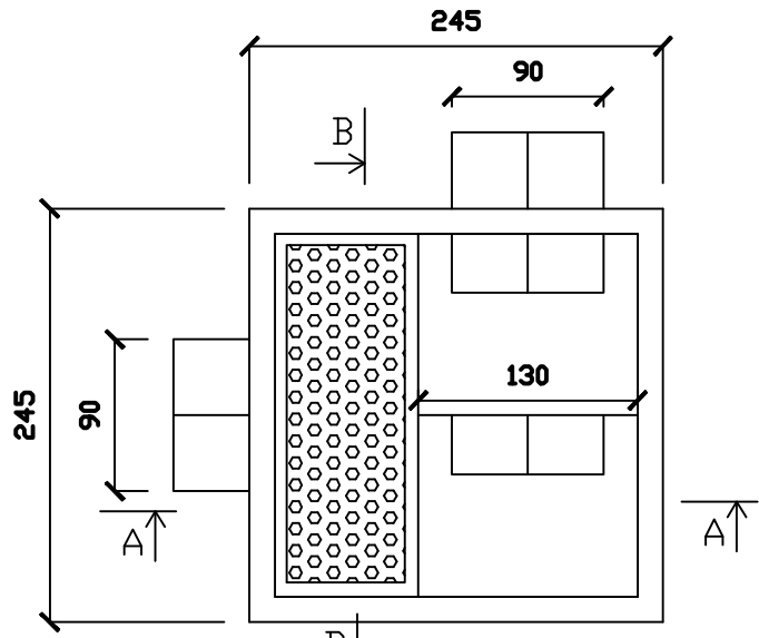
MẶT BẰNG BÈ TÁCH MỠ
